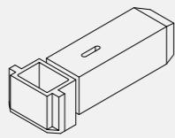
zugeschnittener Eckverbinder
